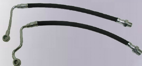
Povratno crevo goriva M12X1,5 L=300mm OZNAKA:300.011
