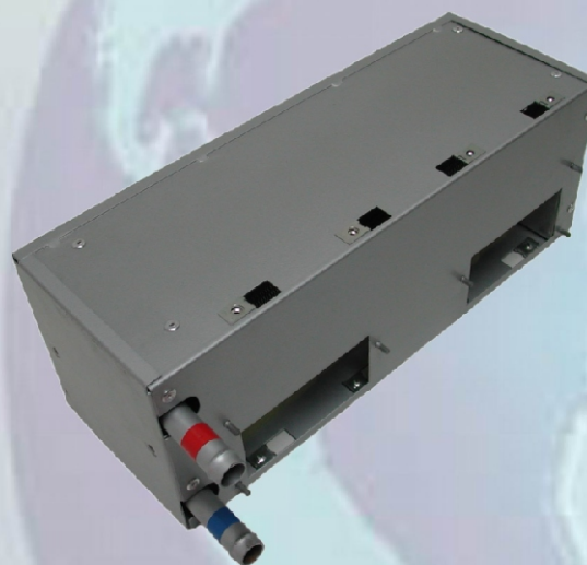
Kučište HERCULES sa grejnim telom, komplet OZNAKA: 2503.01.00
